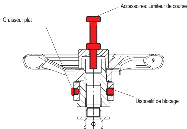
Graisser plat / Dispositif de blocage / Limiteur de course
